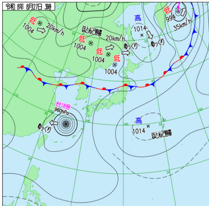
地上天気図 (8月27日3時実況)
