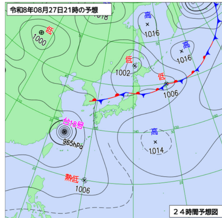
予想天気図 (8月27日21時予想)
