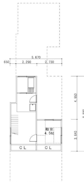
3F 平面図 S1/100
