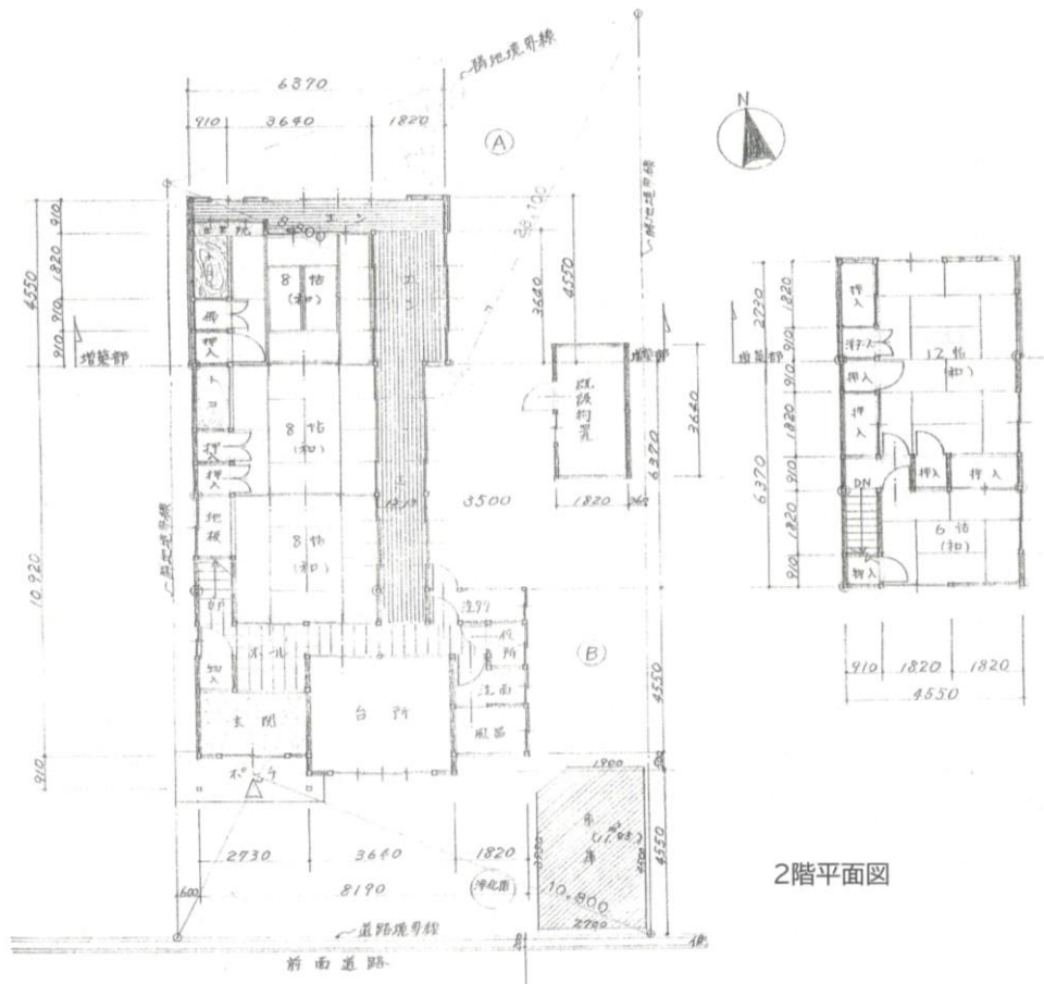
1階平面図
