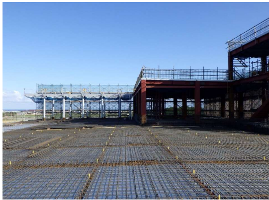
屋上では、床にコンクリートを打つための鉄筋を組み上げました。
