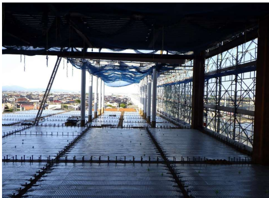
5階部分では、床にコンクリートを打つ準備を進めています。
