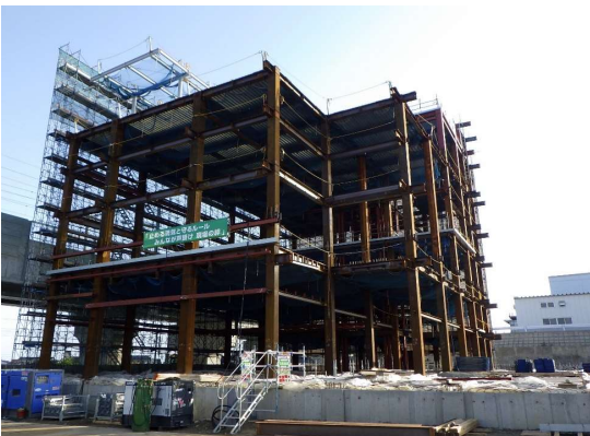
西面（海側）に外部足場が立ちあがりました。
