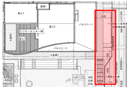
手前：車寄せ屋根 奥：バリアフリー駐車場 基礎型枠、配筋を行いました。
