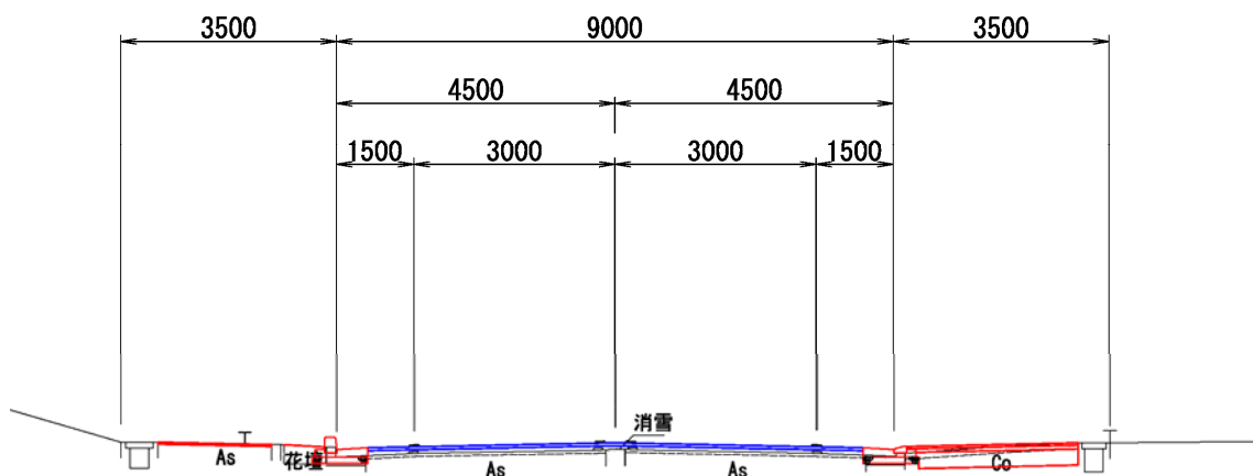
標準断面図
