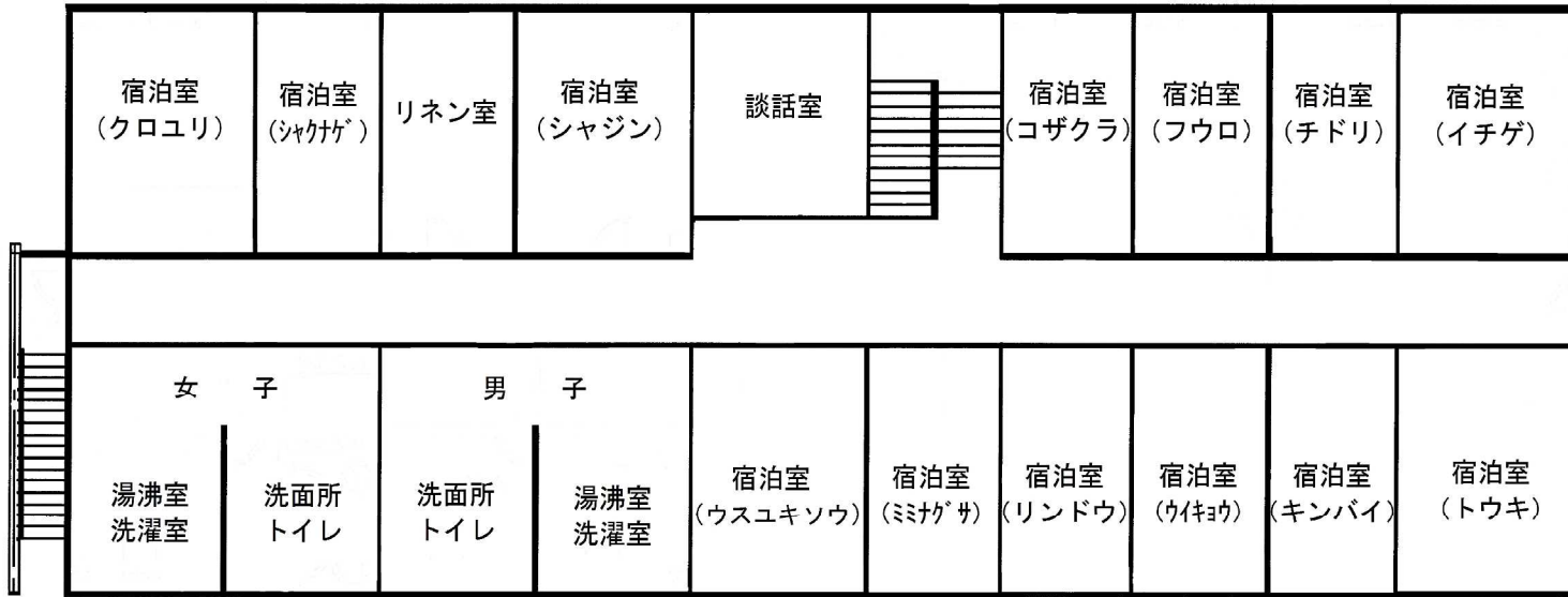
2階平面図
