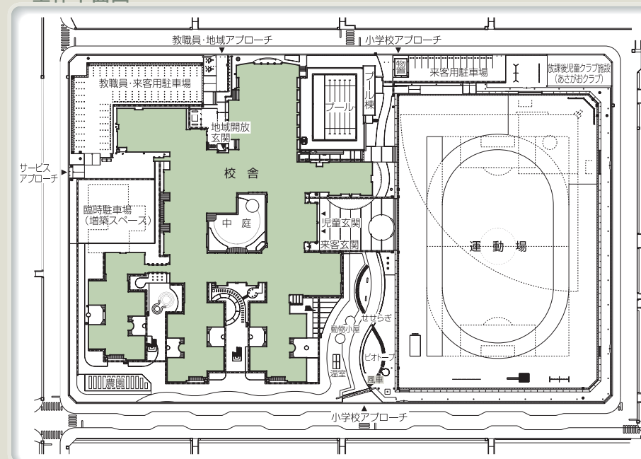
全体平面図
