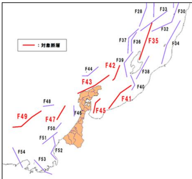
平成28年度津波浸水想定断層位置図
