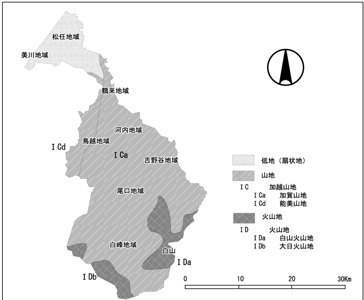
【白山市の地形区分略図】
