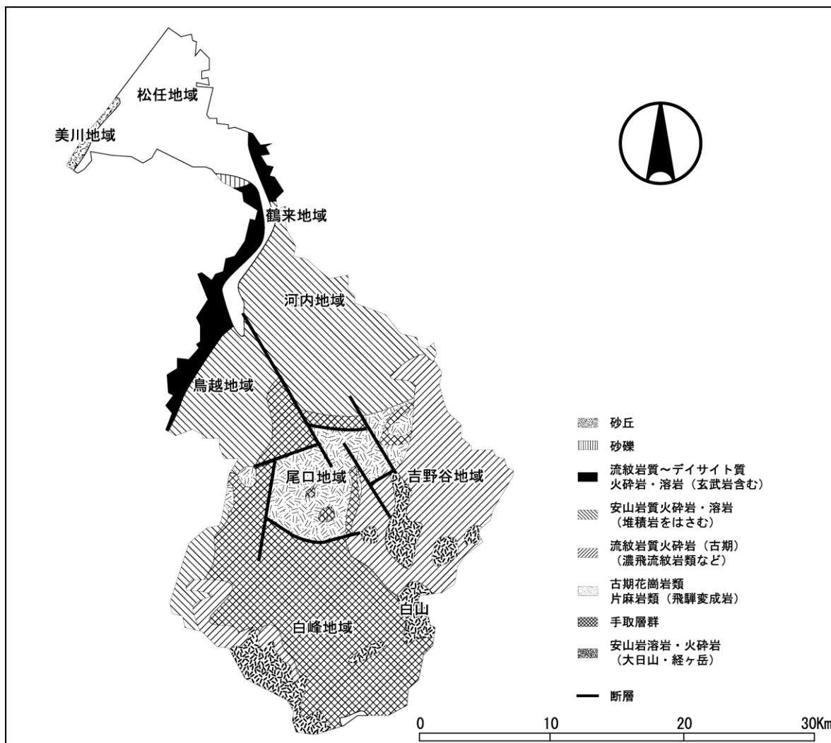
【白山市の地質・地盤分布略図】
